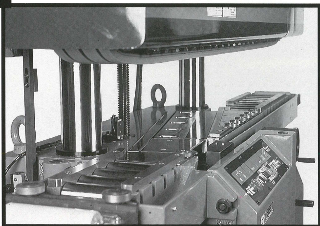
ローラーテーブル(裏刃式) Built-in roller table(Back-knife type)
