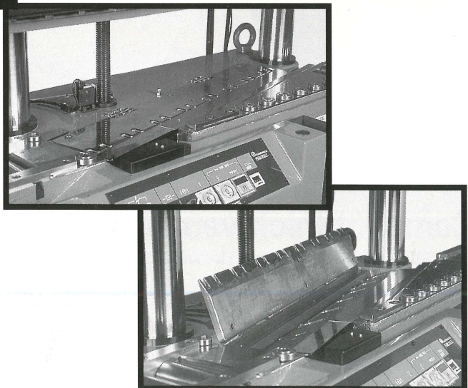
ローラーテーブル(表刃式) Built-in roller table(Knife-Face type)
