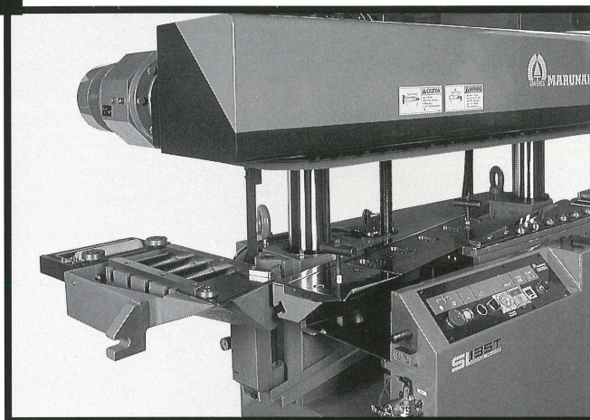
退避リアテーブル(オプション) Retractable rear-table(Option)
