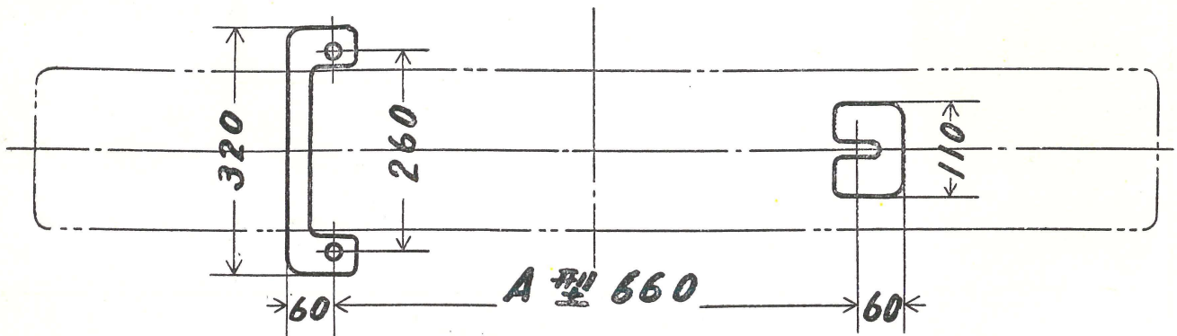
PH "8" A型 (斜刃) 据付図
