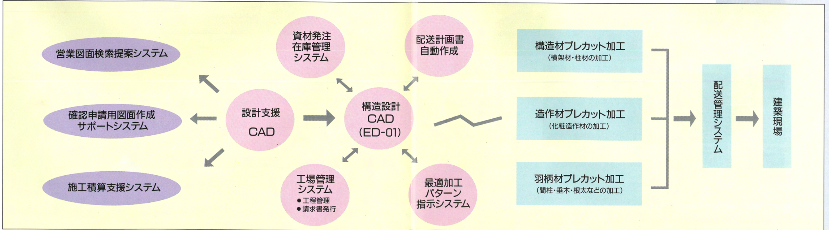
ハイパフォーマンス・プレカット・システム・フロー図
