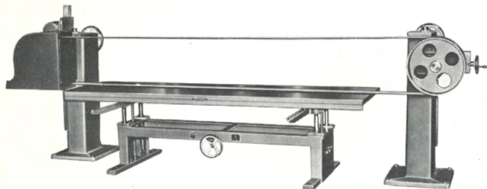
LBP型
