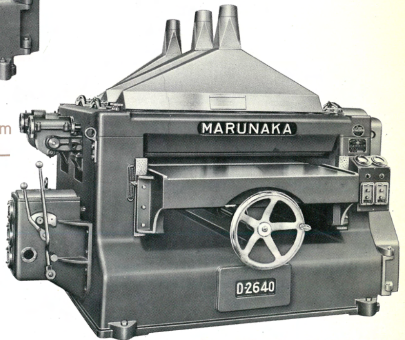
D-2640 1000mm ドラムサンダー
